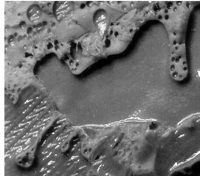
Bondline Void
